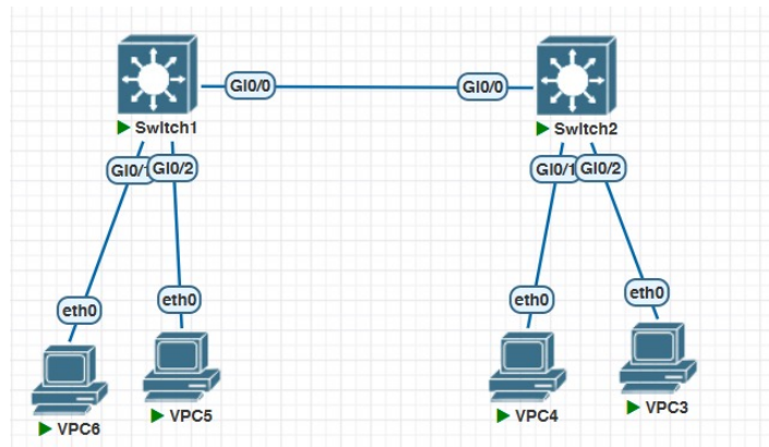
Gambar 1: Topologi Jaringan
